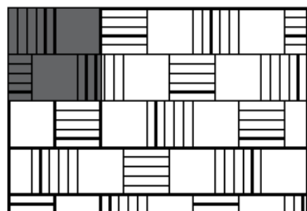
Растер 18 50x50x8cm - 2 броя 50x10x8cm - 10 броя Разход на м 2
