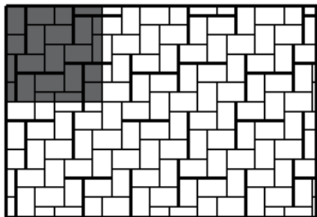
Растер 7 30x20x8cm - 16.68 броя Разход на м 2
