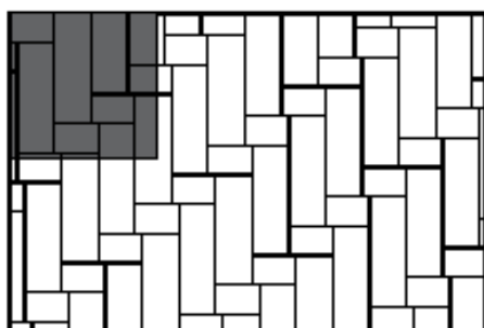
Растер 17 75x25x8cm - 4.03 броя 30x20x8cm - 4.06 броя Разход на м 2
