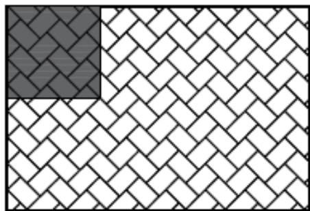
Растер 7 30x20x8cm - 16.68 броя Разход на м 2
