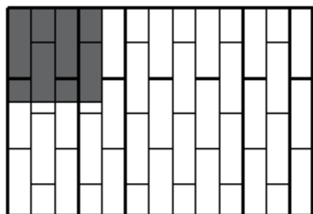
Растер 11 75x25x8cm - 5.34 броя Разход на м 2
