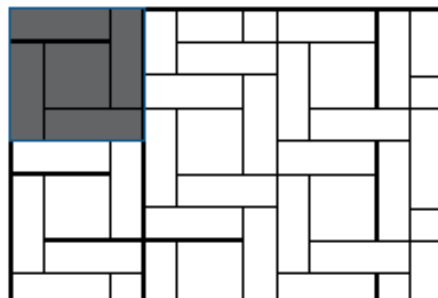
Растер 14 50x50x8cm - 1 броя 50x10x8cm - 4 броя Разход на м 2
