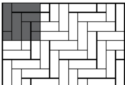
Растер 13 75x25x8cm - 5.34 броя Разход на м 2
