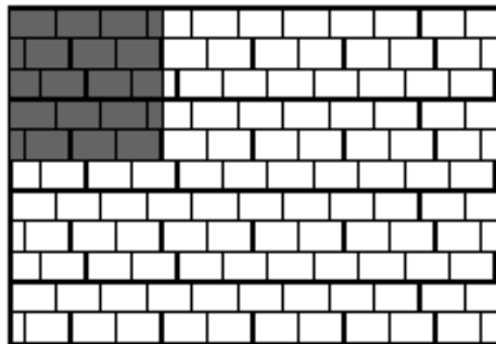
Растер 8 30x20x8cm - 16.67 броя Разход на м 2
